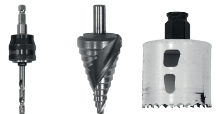
Forets de perçage Foret fraise étagé Scie cloche
